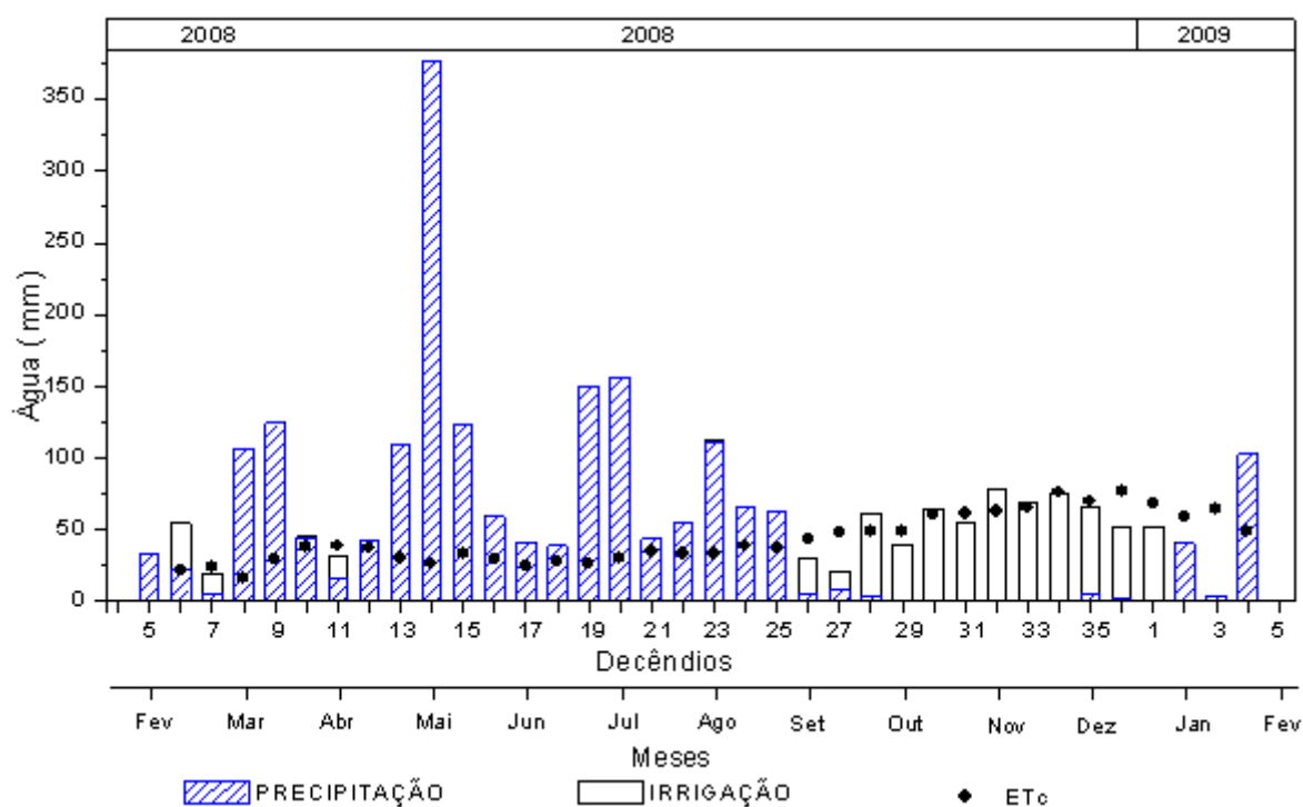
Figura 4. Entrada (precipitação pluvial + irrigação) e saída (evapotranspiração da cultura, ETc) de água no cultivo (2ª folha) de cana-de-açúcar, em Rio Largo – AL, entre os anos 2008-2009.
