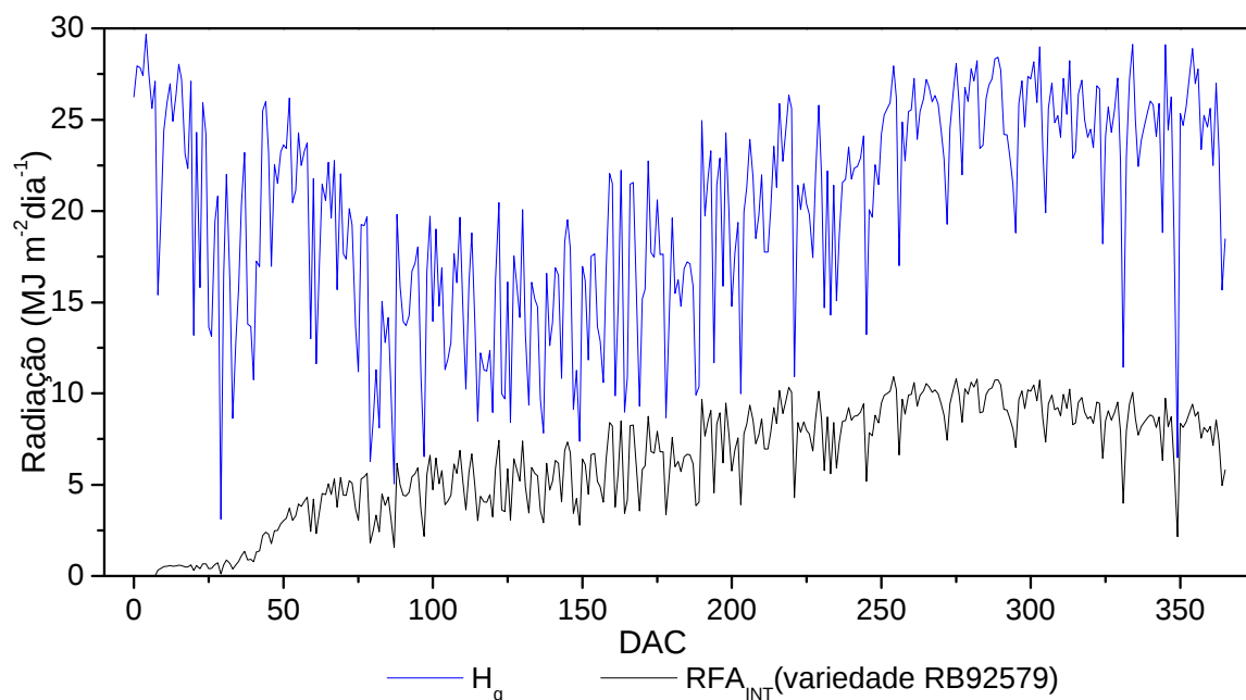
Figura 8. Irradiação solar global diária ( H_g ) e fotossinteticamente ativa interceptada ( \text{RFA}_{\text{INT}} ) da variedade RB92579 em função ao dias após o corte (DAC) durante o ciclo cultura da cana-de-açúcar em Rio Largo – AL, entre 2008 e 2009.
