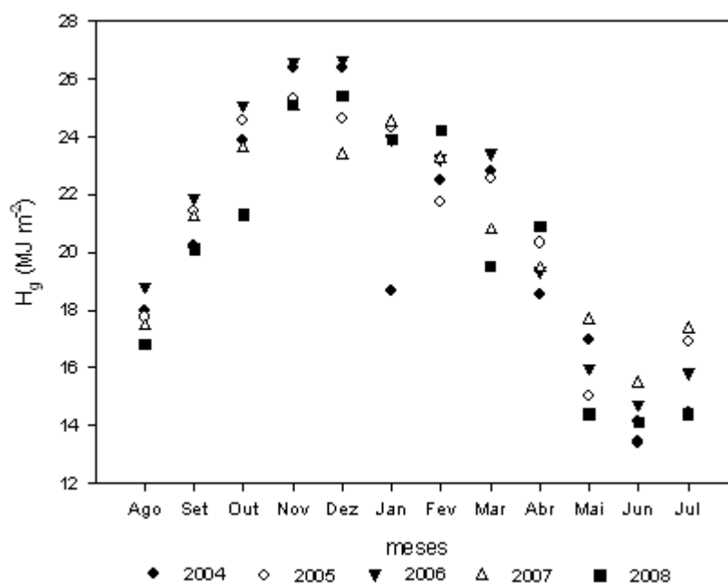
Figura 17. Média mensal da irradiação solar global ( H_g ) da região de Rio Largo, Alagoas.
