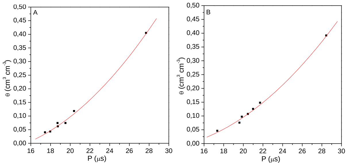
Figura 5. Curva de Calibração da umidade volumétrica do solo ( \theta ) obtida por gravimetria em relação ao período ( P ) da onda do refletômetro em micro segundos. A) profundidade de 0,0 m a 0,30 m e B) profundidade de 0,30 m a 0,60 m.
