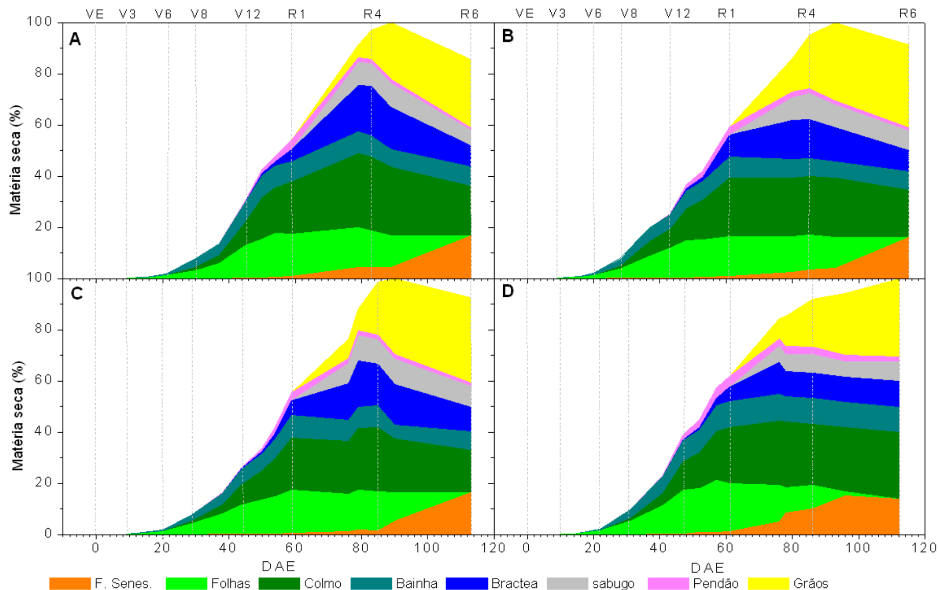
Figura 11. Matéria seca acumulada por partes da planta em % do total, em função dos estádios fenológicos (VE a R6) e dias após a emergência (DAE), para as quatro épocas de semeadura, [T1 06/05/08 (A), T2 19/05/08 (B), T3 10/06/08 (C) e T4 30/06/08 (D)].
