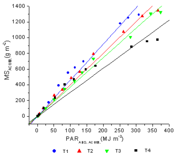
Figura 15. Relação entre a produção de massa seca acumulada total (MS, g m -2 ) do milho e a radiação fotossinteticamente ativa absorvida acumulada (RFA abs , MJ m -2 ), semeado em quatro épocas: tratamento T1 ( y = 4,61x , r^2 = 0,99 ), tratamento T2 ( y = 4,03x , r^2 = 0,99 ), tratamento T3 ( y = 3,74x , r^2 = 0,99 ), tratamento T4 ( y = 2,98x , r^2 = 0,98 ), na região de Arapiraca-AL.
