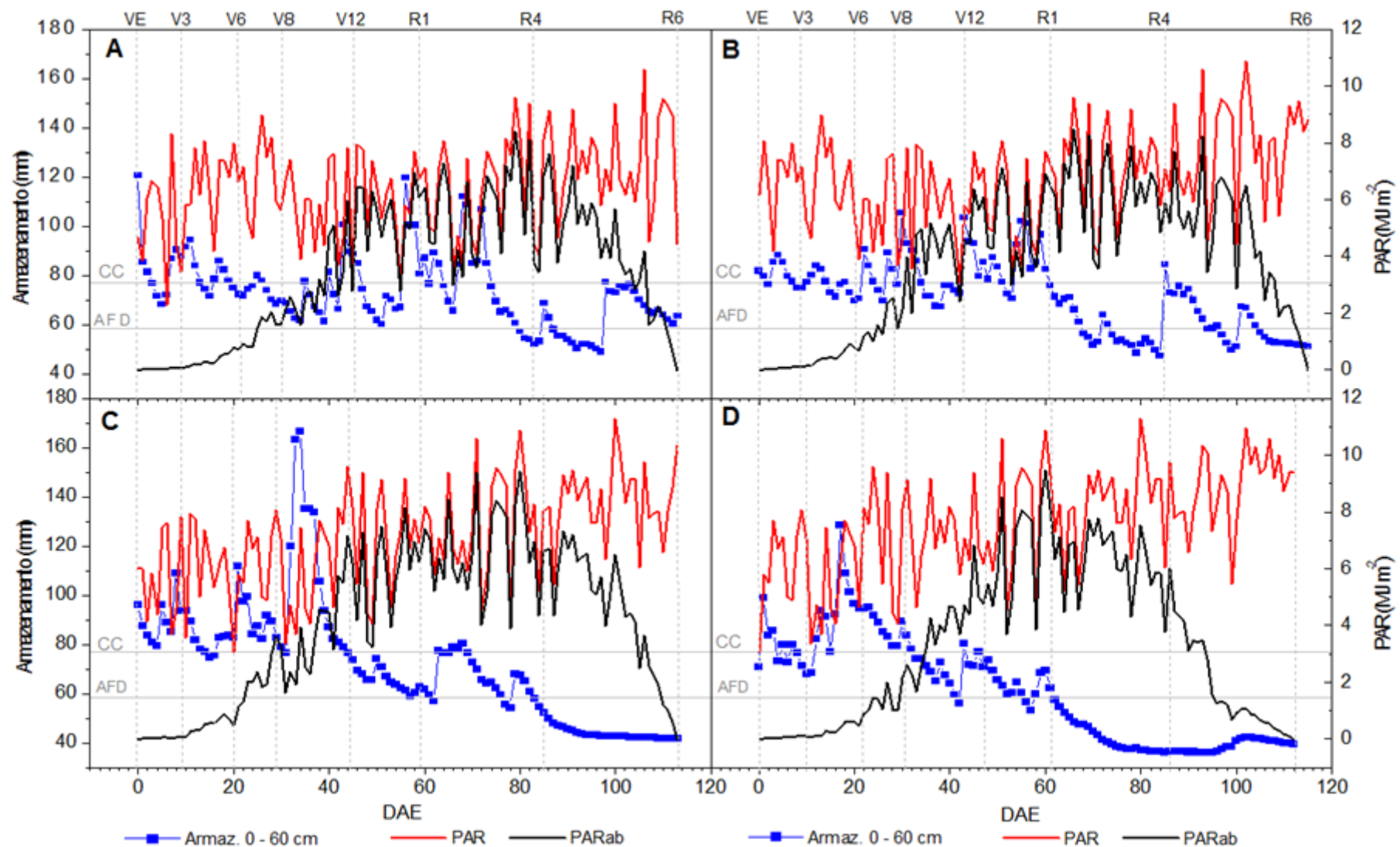
Figura 10. Armazenamento de água no solo (mm), RFA e RFA abs (MJ m -2 ), em função dos dias após a emergência (DAE) para quatro épocas de semeadura de milho [T1 06/05/08 (A), T2 19/05/08 (B), T3 10/06/08 (C) e T4 30/06/08 (D)].
