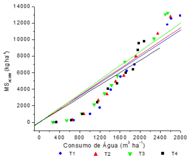
Figura 14. Relação entre a produção de massa seca acumulada total (MS, kg ha -1 ), e o consumo de água (m 3 ha -1 ), do milho semeado em quatro épocas: tratamento T1 (y = 3,98x, r 2 = 0,95), tratamento T2 (y = 4,09x, r 2 = 0,97), tratamento T3 (y = 4,28x, r 2 = 0,96), tratamento T4 (y = 3,76x, r 2 = 0,93), na região de Arapiraca-AL
