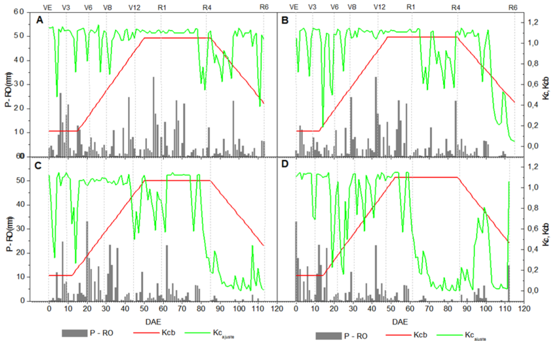
Figura 8. Coeficiente de cultura basal ( K_{cb} ), coeficiente de cultura ajustado ( K_{c\_ajuste} ) e precipitação pluvial menos o escoamento superficial ( P-RO ) em função dos dias após a emergência (DAE) e dos estádios fenológicos do milho (VE a R6) para quatro épocas de semeadura de milho [T1 06/05/08 (A), T2 19/05/08 (B), T3 10/06/08 (C) e T4 30/06/08 (D)].
