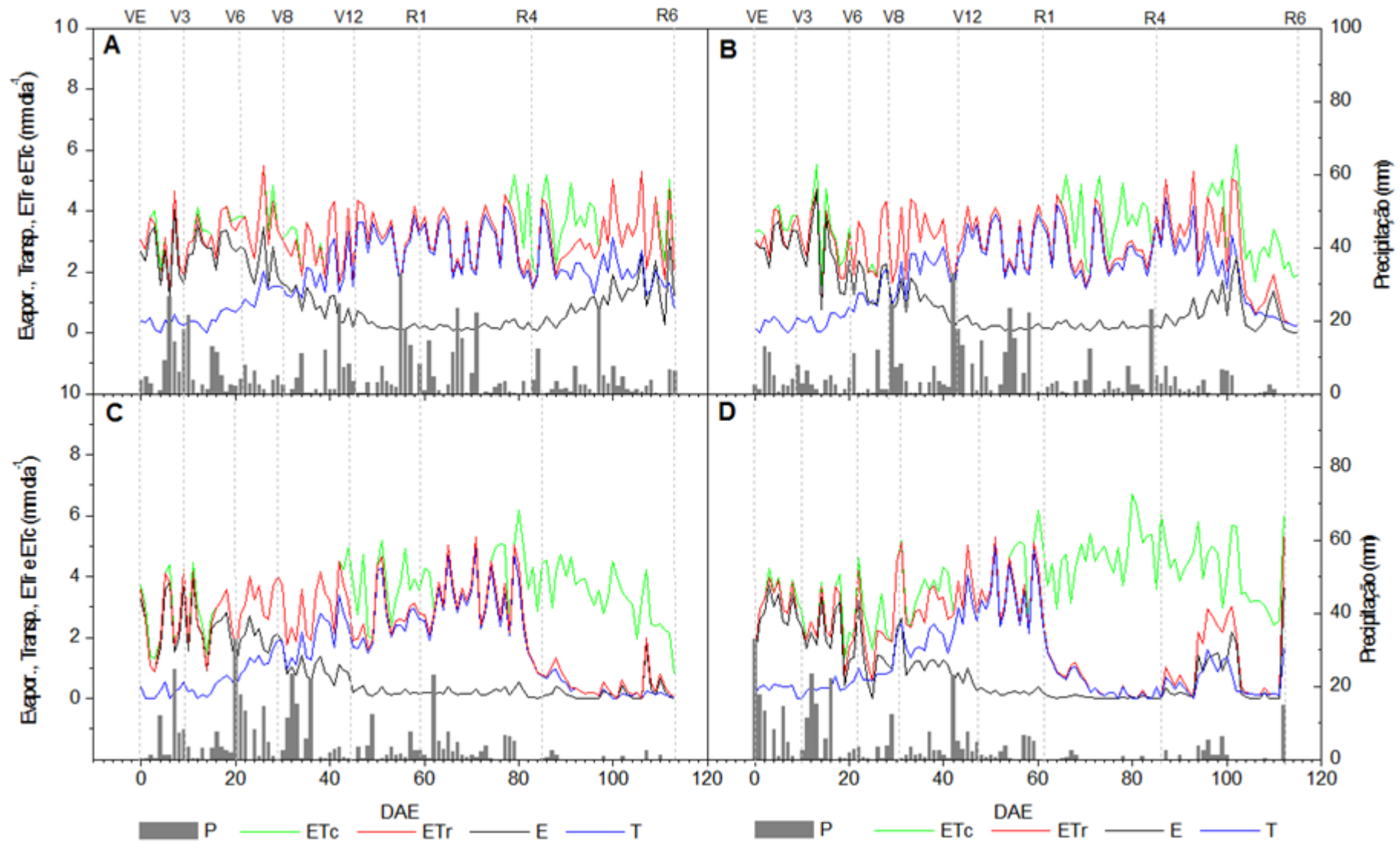
Figura 9. Precipitação pluvial (P), evapotranspiração da cultura ( ET_c ), evapotranspiração real ( ET_r ), Evaporação (E) e transpiração (T) para quatro épocas de semeadura [T1 06/05/08 (A), T2 19/05/08 (B), T3 10/06/08 (C) e T4 30/06/08 (D)].
