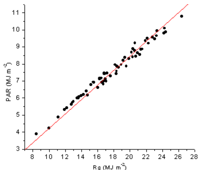
Figura 6. Relação entre a radiação fotossinteticamente ativa (RFA, MJ m -2 ) e Radiação global (Rg, MJ m -2 ) ( y = 0,423 (\pm 0,0017)x , r^2 = 0,99 ), na região de Arapiraca-AL.
