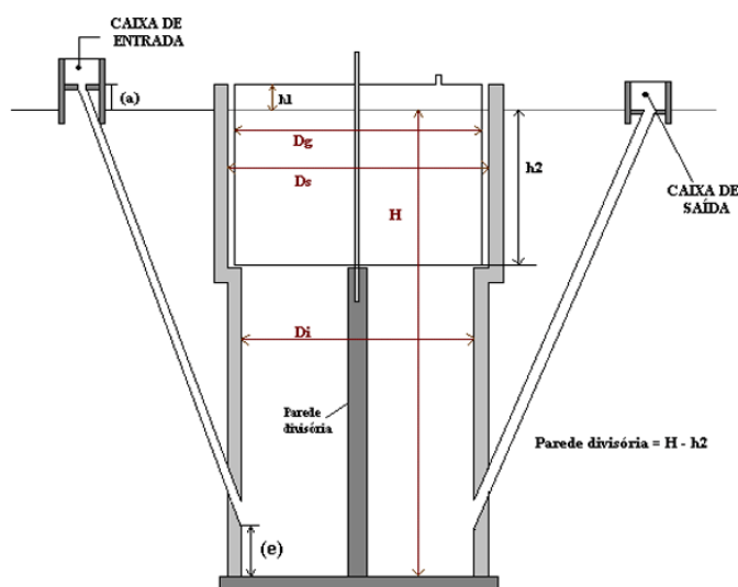
Figura 7: Biodigestor Indiano
