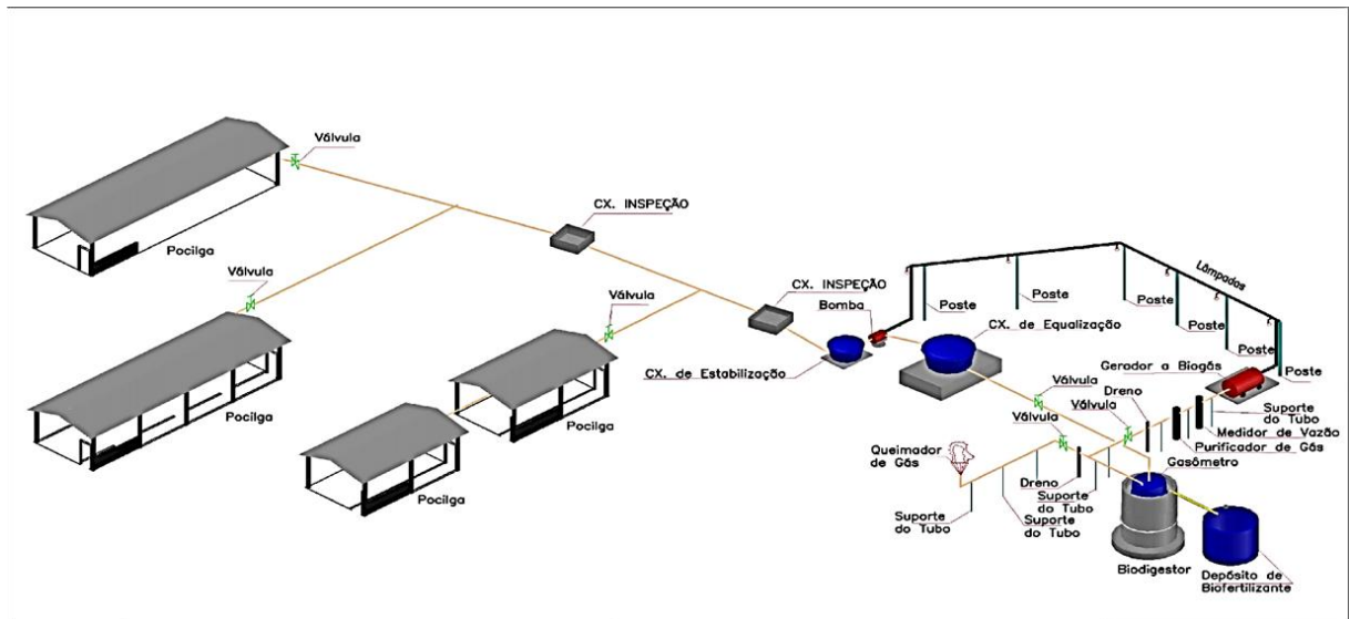
Figura 19: Esquema de Alimentação do Biodigestor
