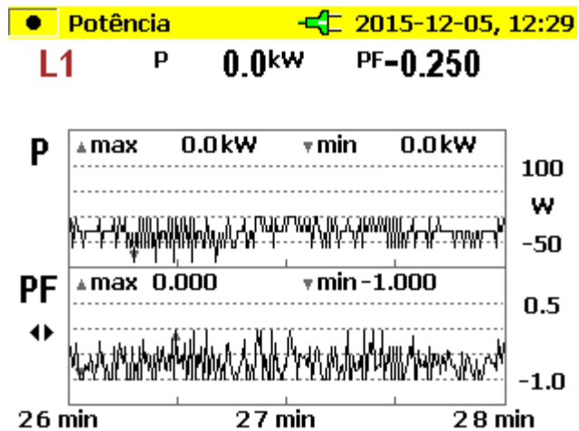
Figura 33: Variação do Fator de Potência
