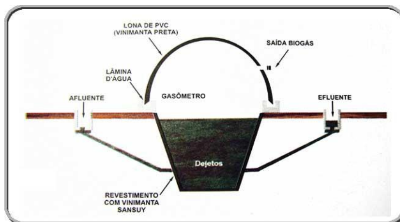
Figura 9: Biodigestor de Lona
