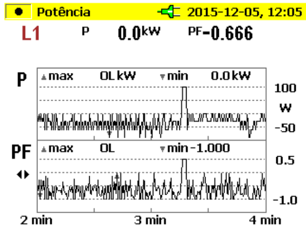
Figura 31: Variação do Fator de Potência
