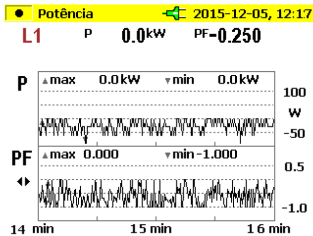
Figura 32: Variação do Fator de Potência
