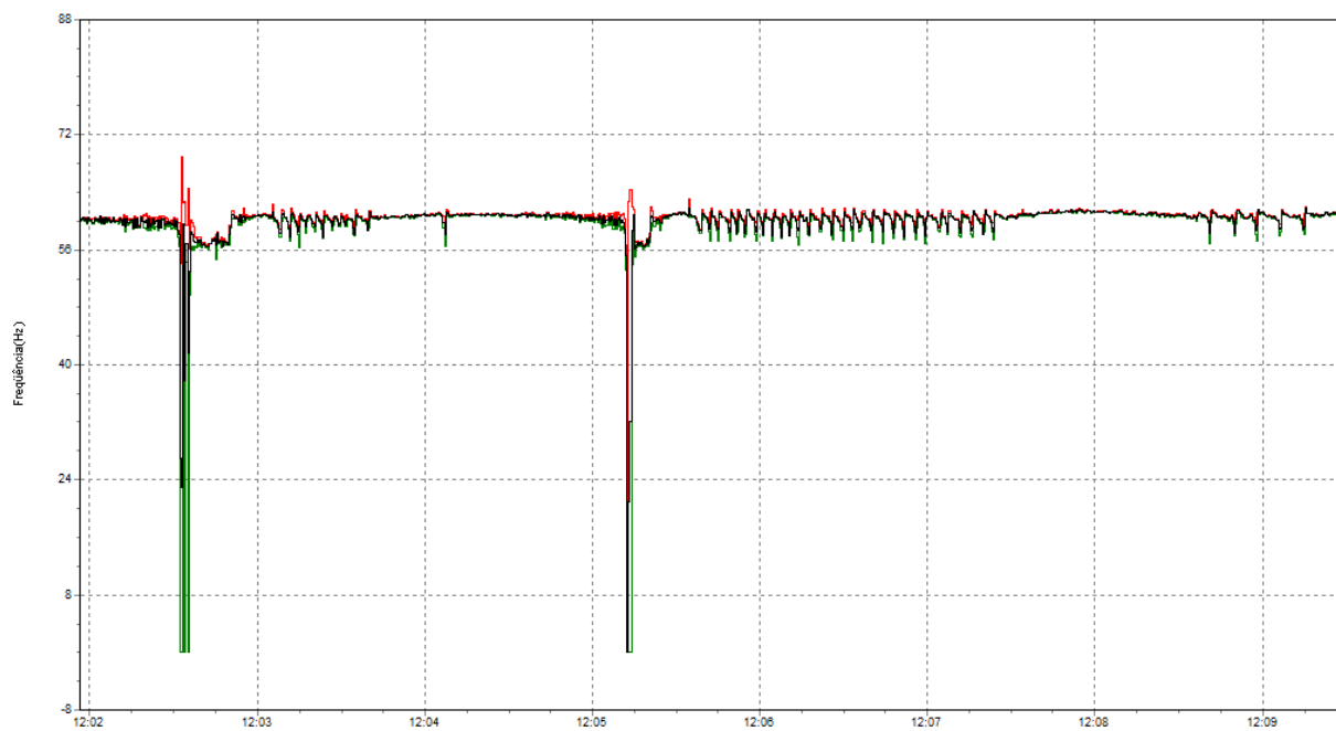
Figura 29: Gráfico da Oscilação da Frequência
