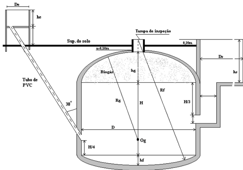
Figura 8: Biodigestor Chinês
