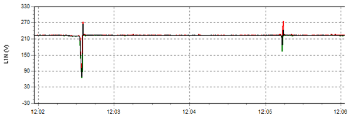
Figura 26: Gráfico do Comportamento da Tensão Elétrica
