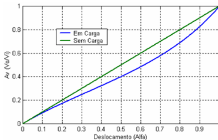
Figura 1: Carga Linear e não linear
