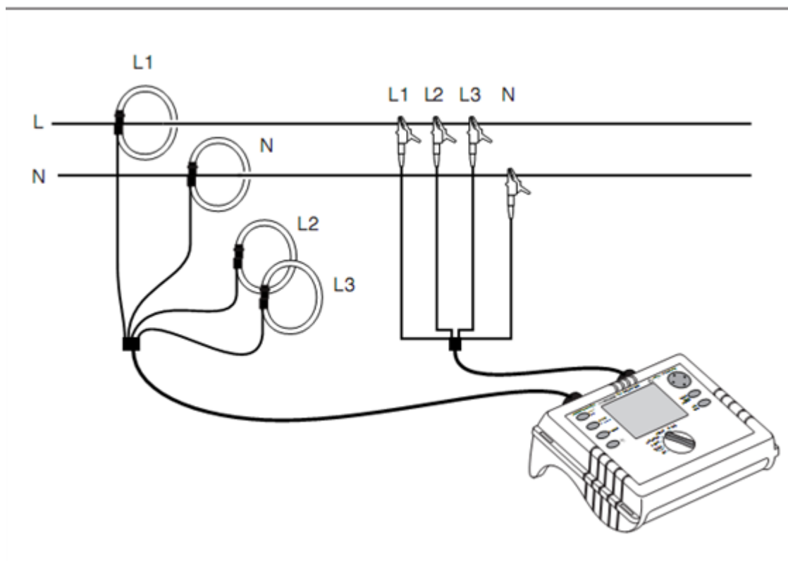
Figura 23: Esquema de Ligação Monofásica do Registrador
